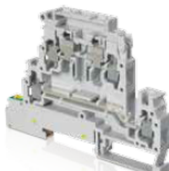
Двухуровневные клеммы - Для предохранителей 5 x 20 mm и 5 x 25 mm (0.197" x 0.787" и 0.197" x 0.984")
