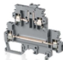
Отключение с помощью ножевого контакта
